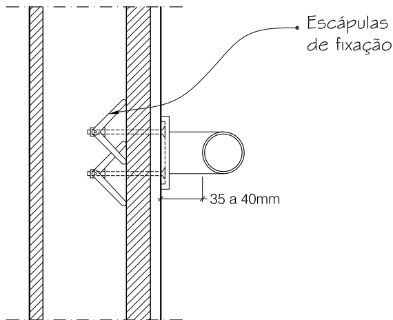
E Tipo de parede oca
