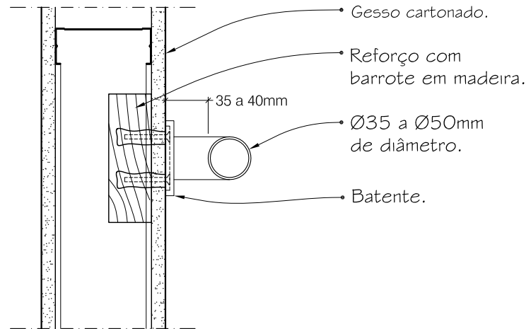
D Reforço interior de divisória (gesso cartonado)
