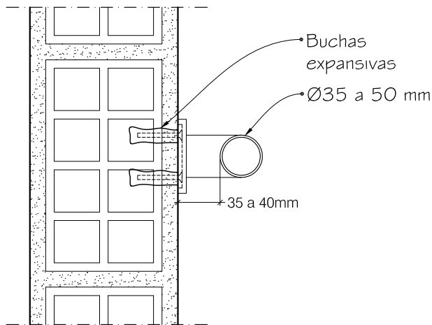
C Parede em alvenaria de tijolo de 11cm
