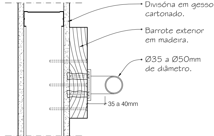
F Reforço exterior de divisória
